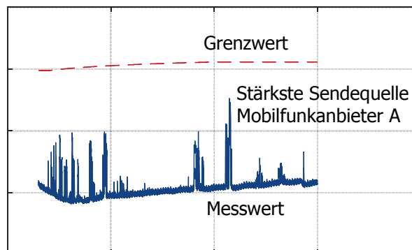
Bild 2: Spektrum am Ort der maximalen Feldstärke.
